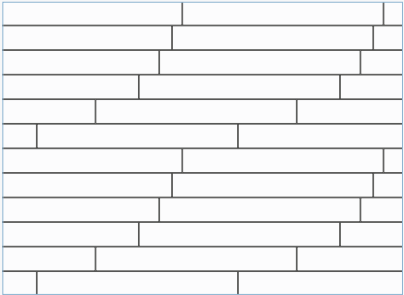
Regular laying (sequence/secuencia: 1-3-4, 3-6-7, 3-9-12 cm.) Colocación regular
